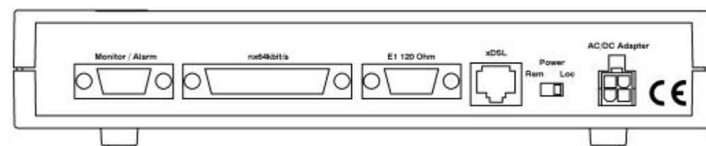
Мультисервисный модуль E1 120 Ом и n x 64 Кбит/с
