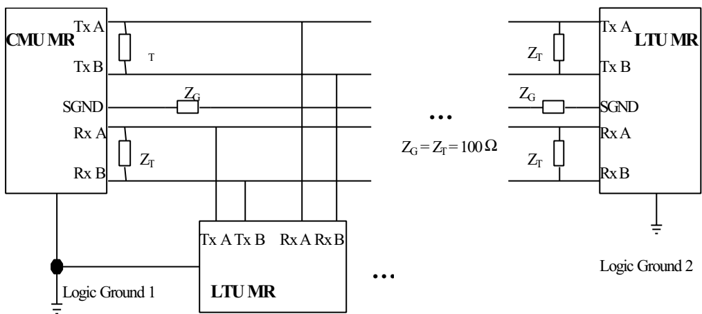
Рисунок 3-16: Согласованная нагрузка для протяженной шины TMN.
