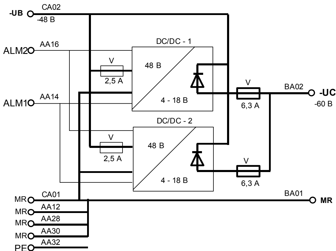
Блок-схема конвертора
