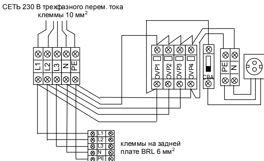
Блок-схема блока распределения трехфазного переменного тока
