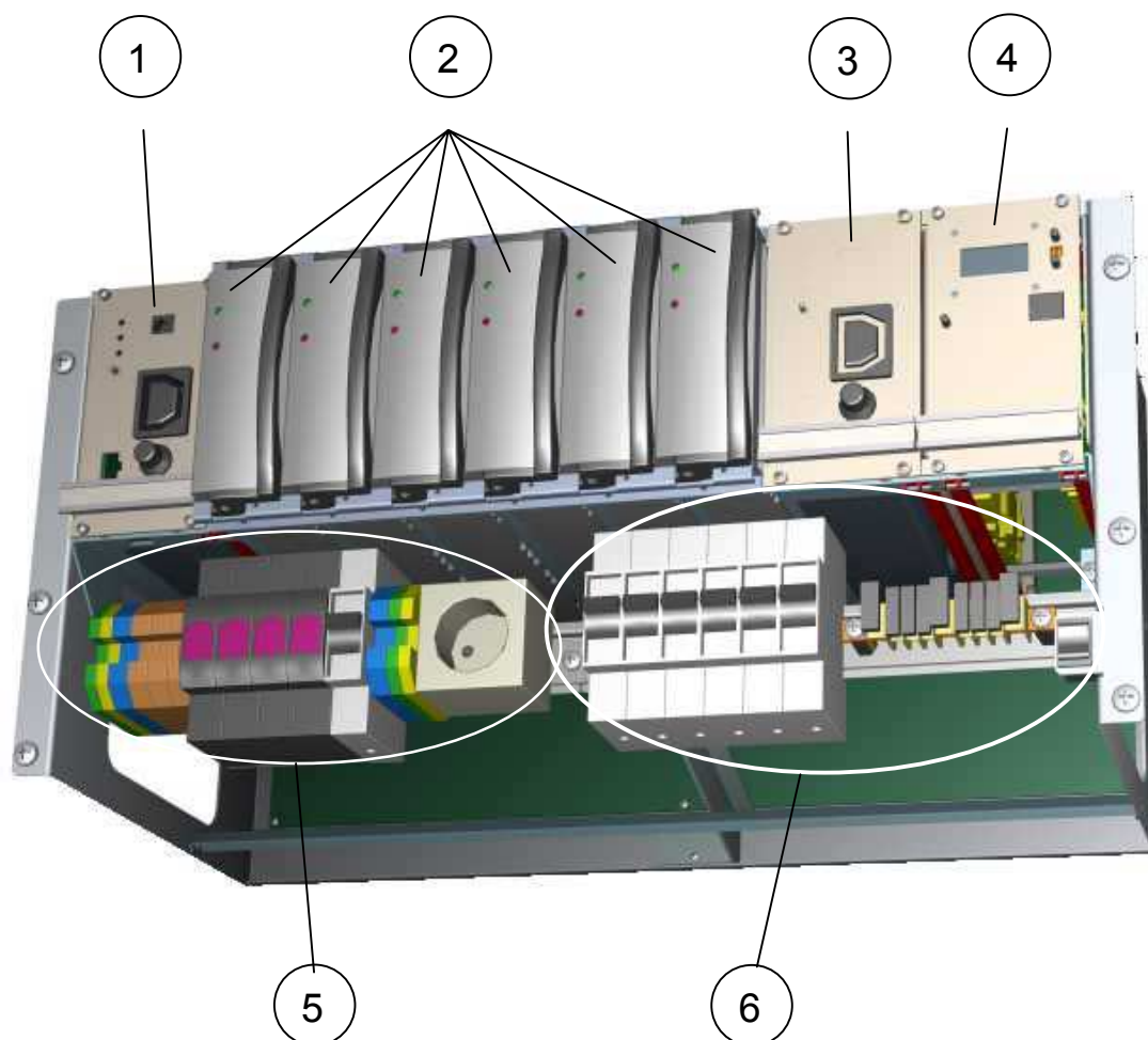
Основная секция MRL системы электропитания MPS
