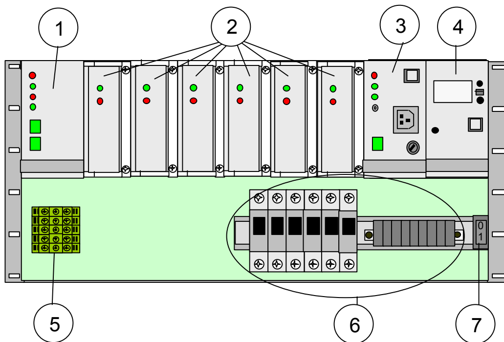
Секция с дополнительным вольтдобавочным конвертором, непосредственное подключение
