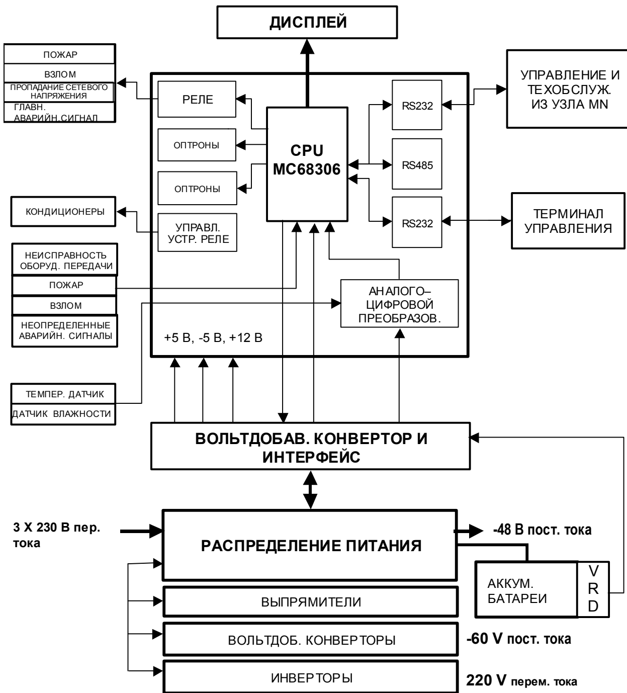
Блок-схема системы MPS и соединения с окружением
