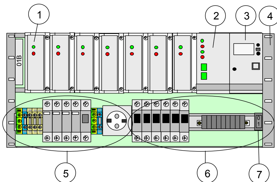
Секция с максимальным количеством выпрямителей, трехфазное подключение
